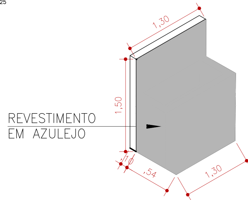
DETALHAMENTO TANQUE EXTERNO Escala: 1/25
