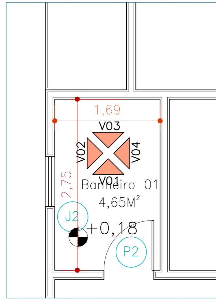
DETALHAMENTO BANHEIRO 01 Escala: 1/25
